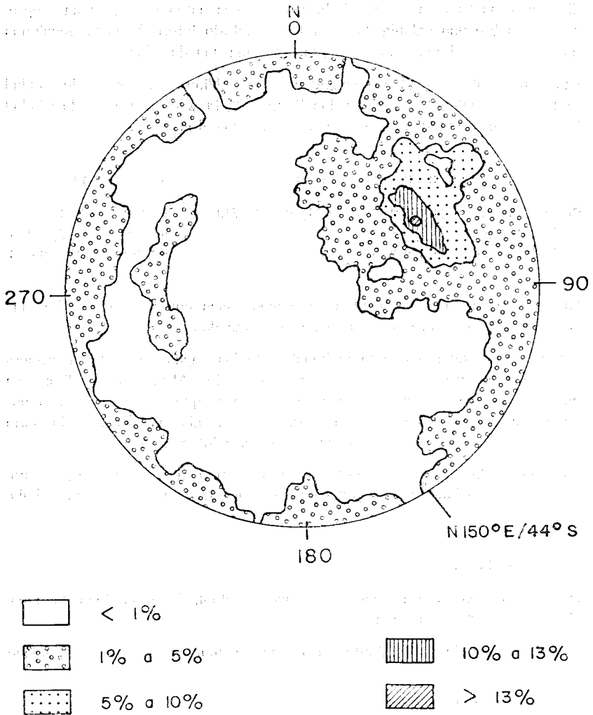
Figura 9.—Proyección de 145* polos de la esquistosidad primaria S_1 Falsilla de Schmidt (Hemisferio Inferior).
