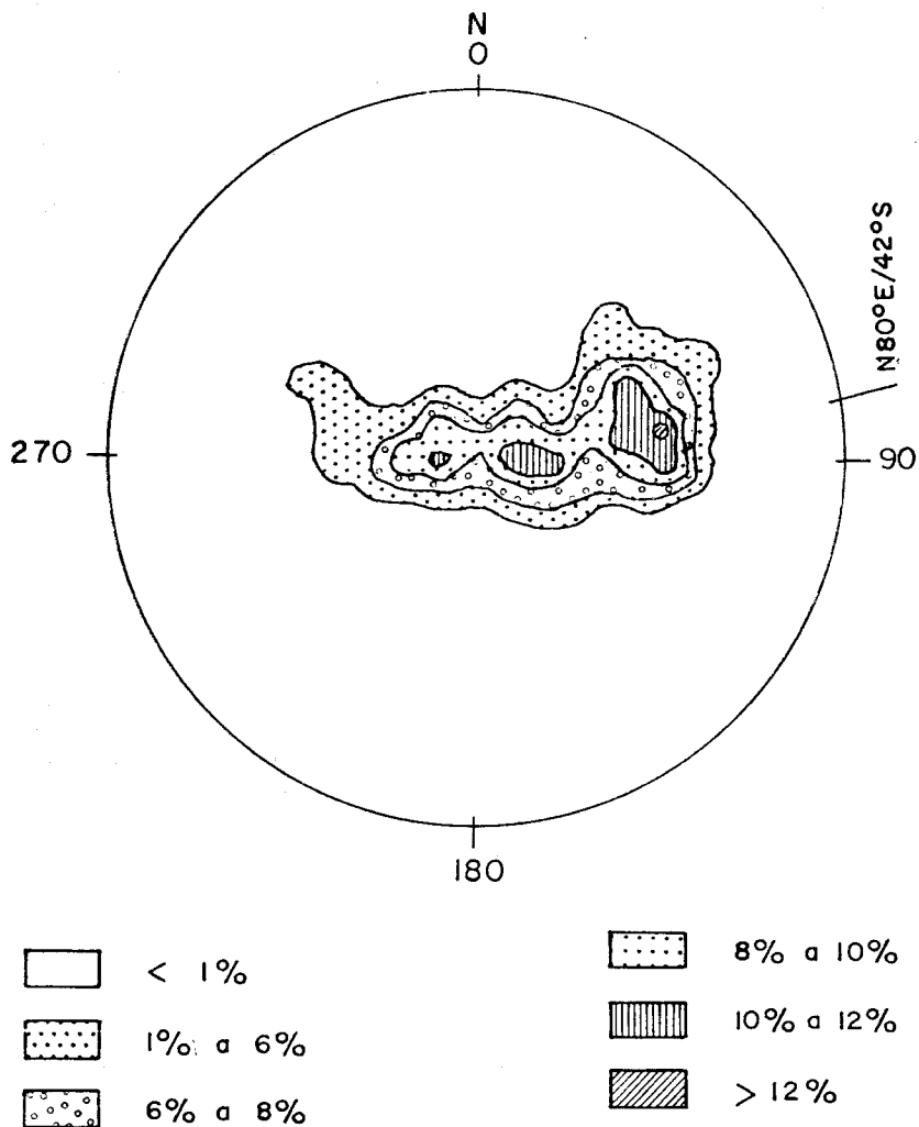
Figura 20.—Proyección de 48 polos de la lineación de intersección L_2 ( S_0S_2 ). Falsilla de Schmidt (Hemisferio Inferior).
